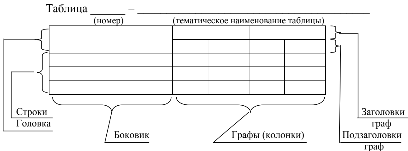
Рисунок 2.6 – Структура таблицы
